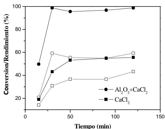
Figura 2. Evolución de la conversión de xilosa (■, ●) y rendimiento en furfural (□, ○) con el tiempo de reacción (175 °C y rel. mástica xilosa:catalizador= 3:1).
