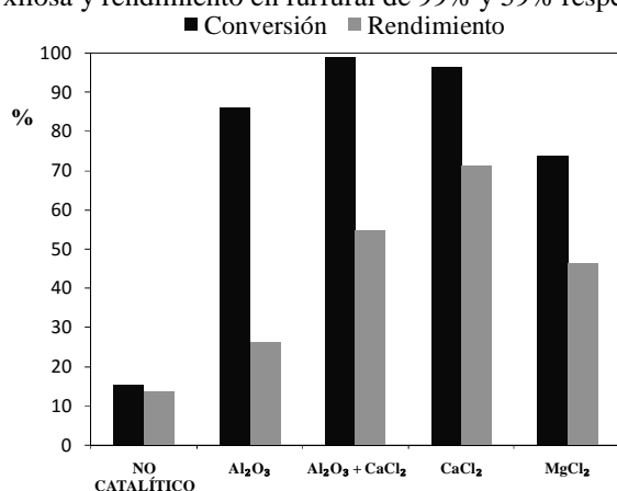
Figura 1. Influencia de la adición de sales, CaCl 2 y MgCl 2 , al medio de reacción (175 °C, 50 min y rel. mástica xilosa:catalizador= 3:1).
