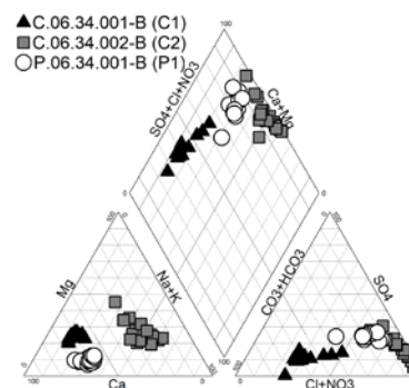
Fig. 2. Diagrama de Piper
