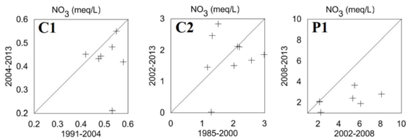
Fig. 4.- Gráficas de Ozgur para nitratos
